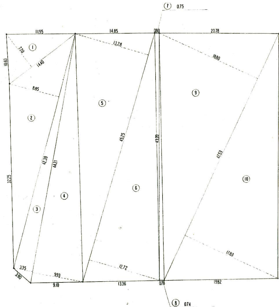
敷地求積図 S=1:200
