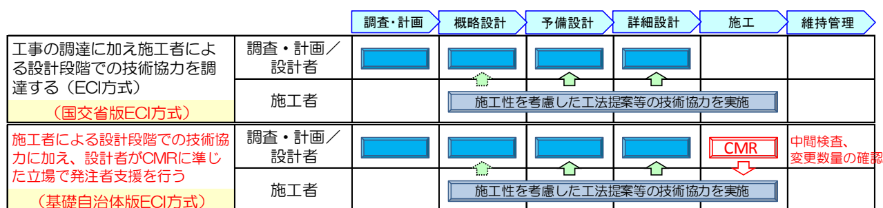
図 4 国交省版 ECI 方式と基礎自治体版 ECI 方式の事業手順
