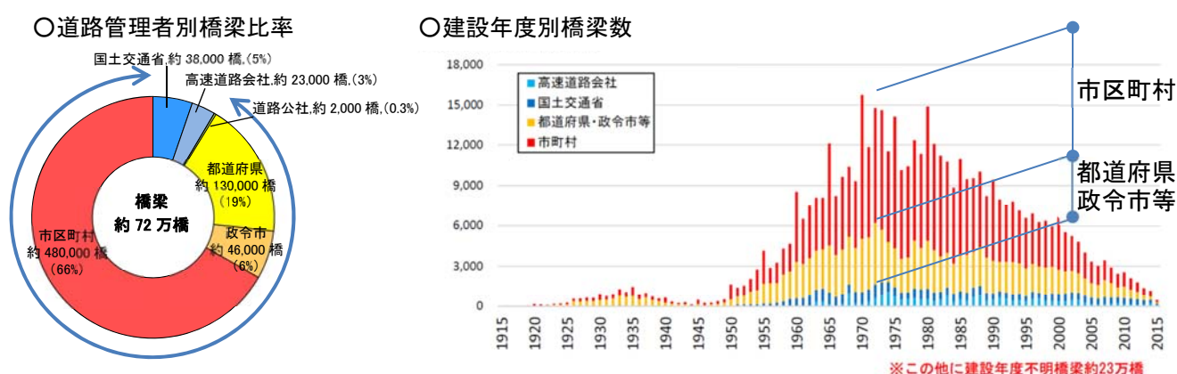
図1 道路管理者別橋梁比率および建設年度別橋梁数（国交省道路局の調査結果 平成 26 年を引用）
