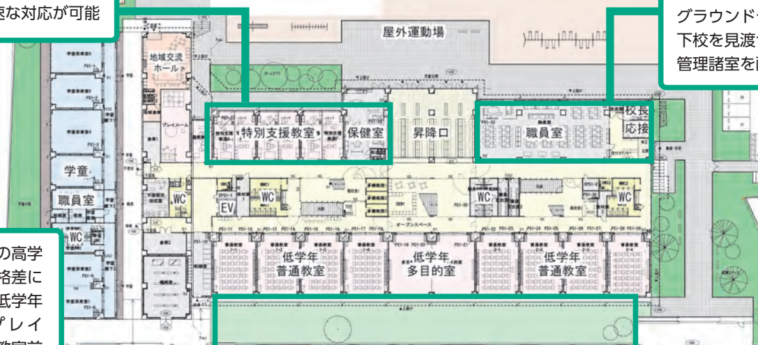
1 階平面図
