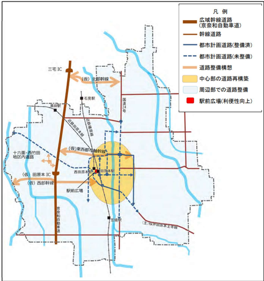
図 3.1 道路・交通の整備方針
